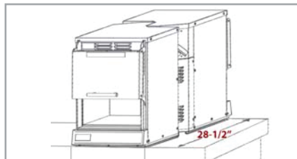
Duas unidades colocadas de costas-para-costas numa prateleira de 28 1/2" (724 mm) em um espaço de 13 5/8" (346 mm)
